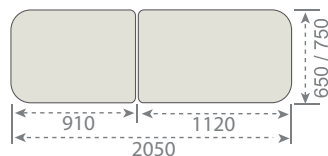
Modèle: ETSXL-B-65/75
