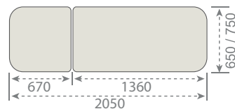
Modèle: ETSL-B-65/75
